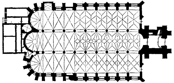
Afb. 1. St.-Martinuskerk, Weert: plattegrond na 1500.
